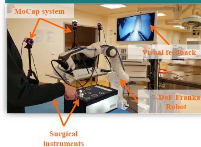
Robot porte caméra pour la CMI
