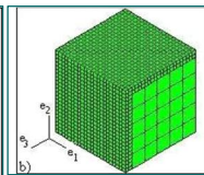
Comparaisons AM (version en transformations finies sans endommagement) / EF. Microstructure périodique soumise à une compression oedométrique selon l'axe e_1 . Matrice viscohyperélastique. Maillage EF d'1/8 de la cellule de base et dilatations axiales dans le grain et les 3 zones intergranulaires [3].
