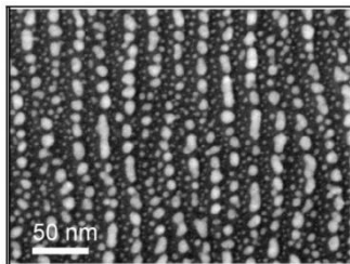
Fig.2 : Micrographie HAADF-STEM de particules d'argent déposées sur une surface d'alumine gravée et recouvertes d'une couche mince d'alumine.
